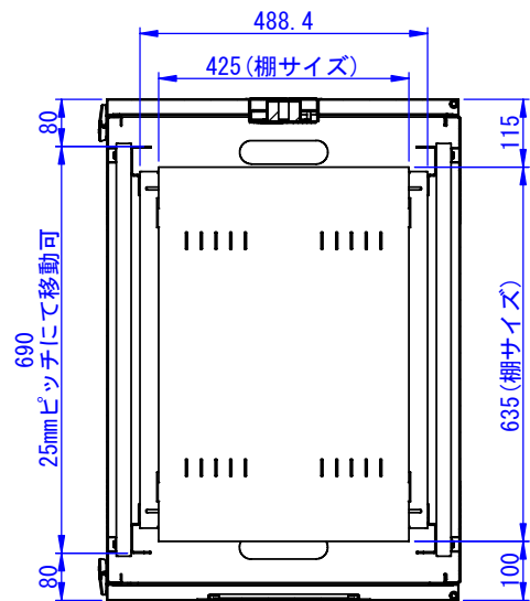
断面図 B-B
