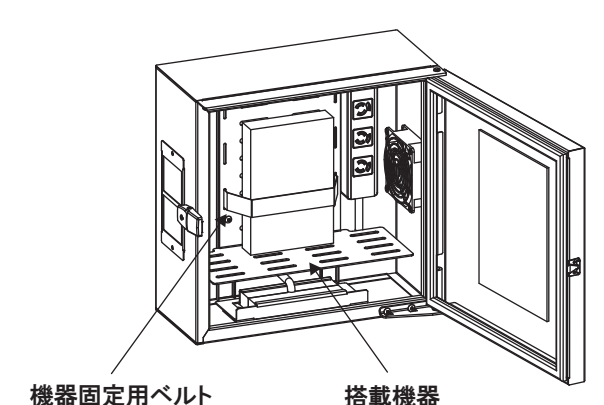
機器+機器固定ベルト設置例 ※機器固定用ベルト別売り
