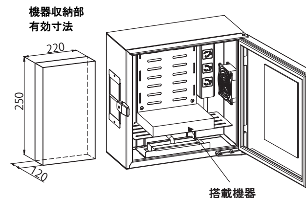
機器設置例
