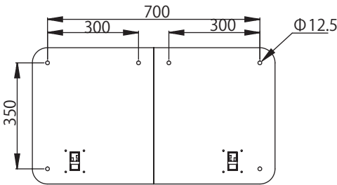
アンカー施工寸法
