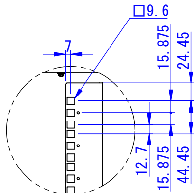
詳細図 B スケール 1 : 5
