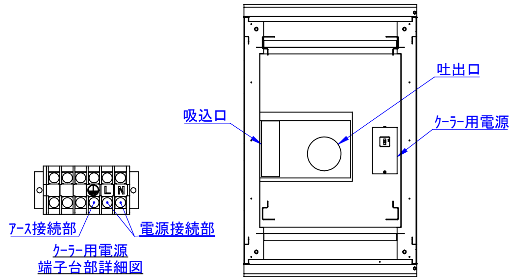
断面図 D-D
