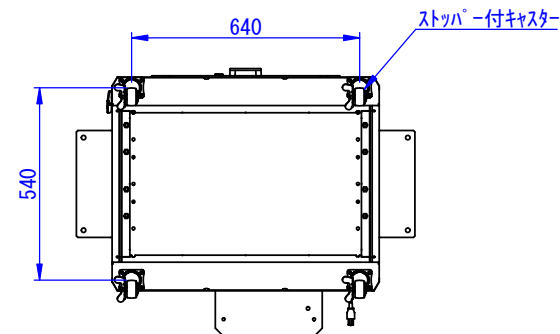
底面図
