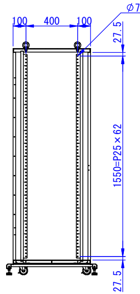
断面図 A-A
