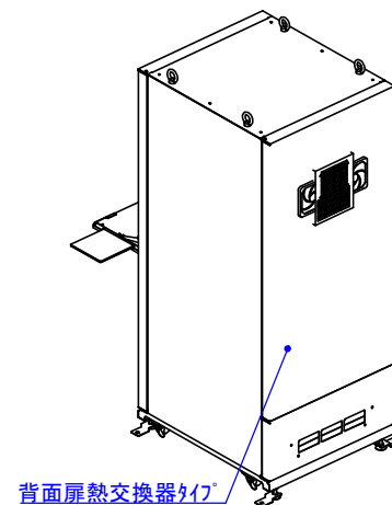
取付イメージ (S15)
