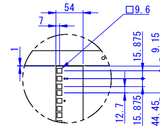
詳細図 C スケール 1 : 5
