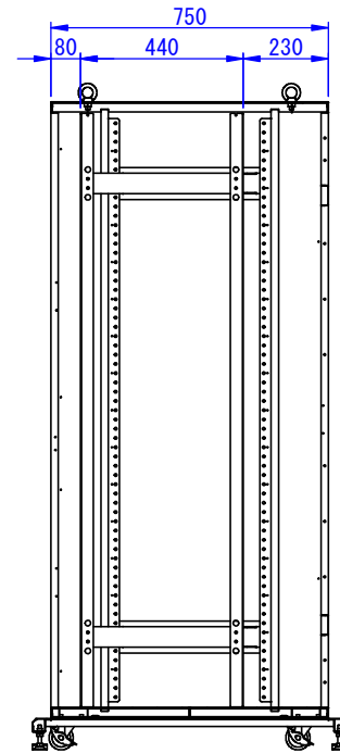
断面図 B-B
