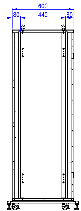
断面図 B-B
