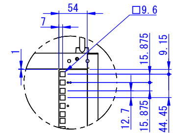
詳細図 C スケール 1 : 5
