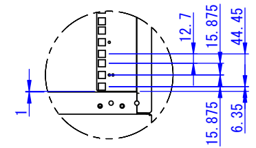
詳細図 D スケール 1 : 5
