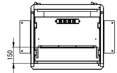
断面図 A-A
