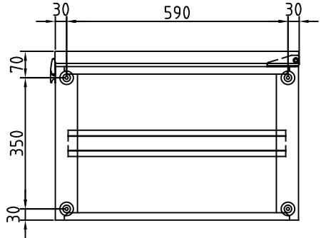
底 面
