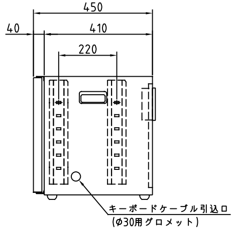
側 面
