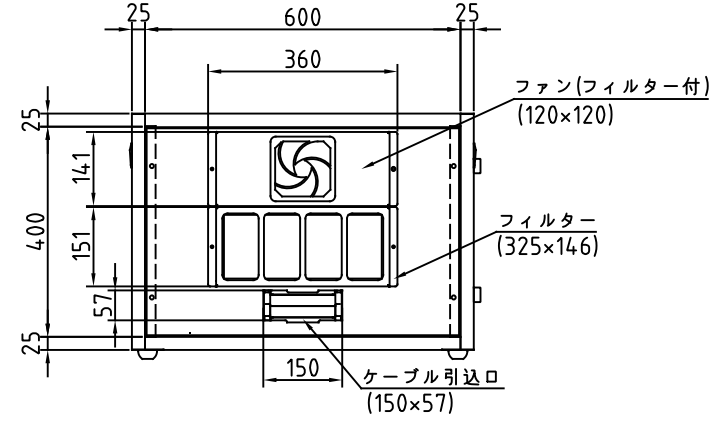
背 面
