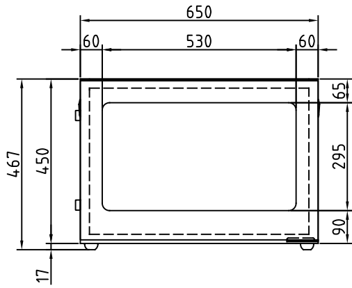
正 面
