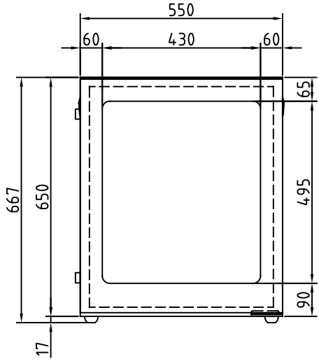
正 面
