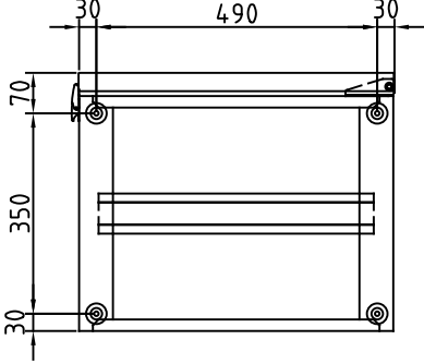
底 面
