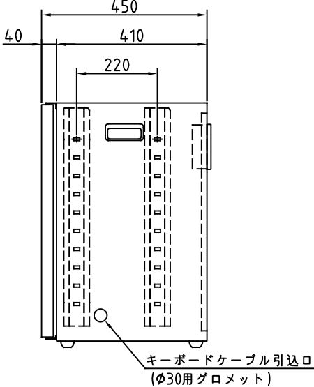
側 面
