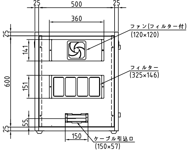
背 面
