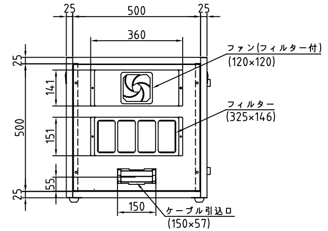
背 面
