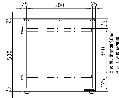
正 面 (扉を外した時)
