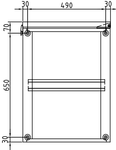
底 面
