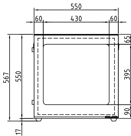
正 面
