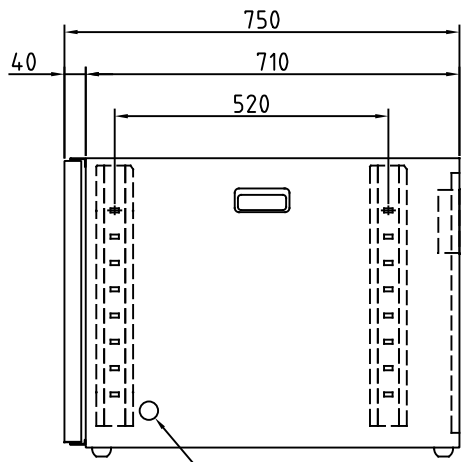
側 面
