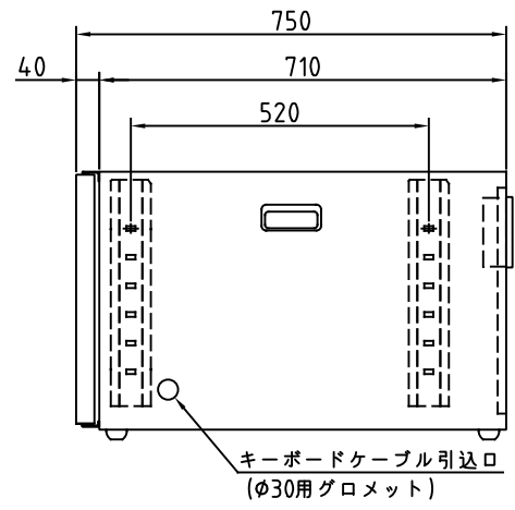
側面
