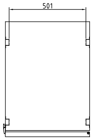
上面
