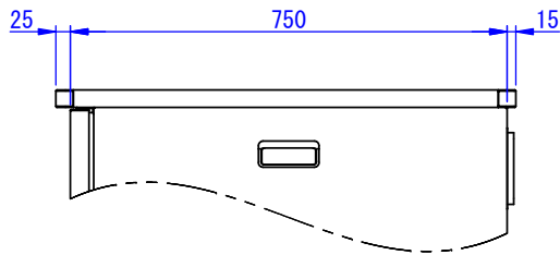
本体組付け側面図
