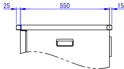
本体組付け側面図
