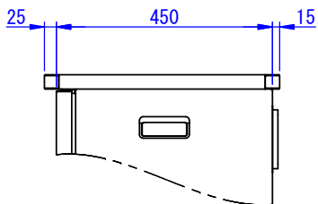
本体組付け側面図
