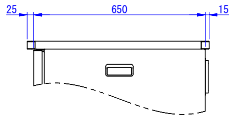
本体組付け側面図
