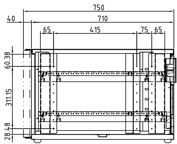
A-A断面図
