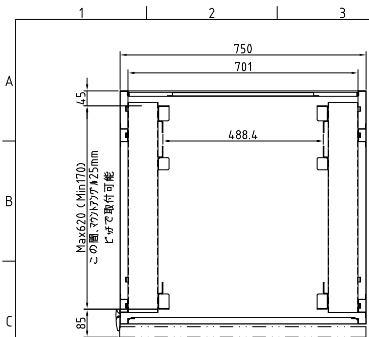
B-B断面図
