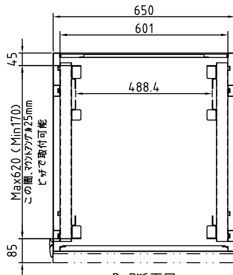
B-B断面図
