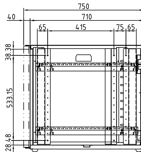
A-A断面図
