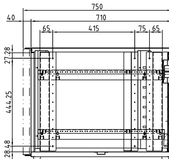
A-A断面図
