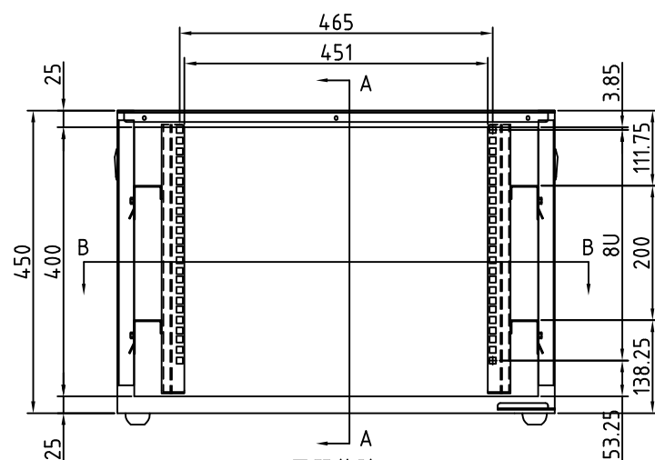
扉開放時
