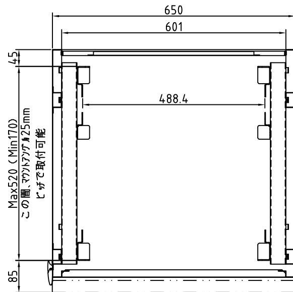
B-B断面图
