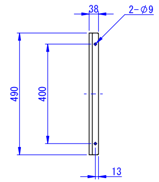
ディスプレイケース取付金具詳細
