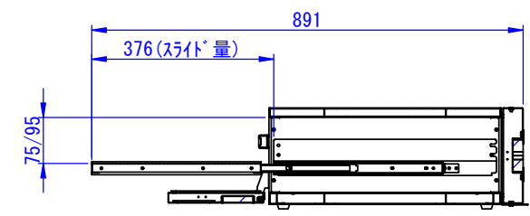
本体取付イメージ スケール: 1:10
