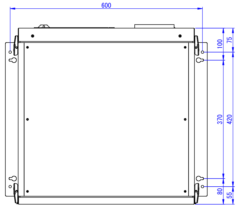
本体取付イメージ(上面図)
