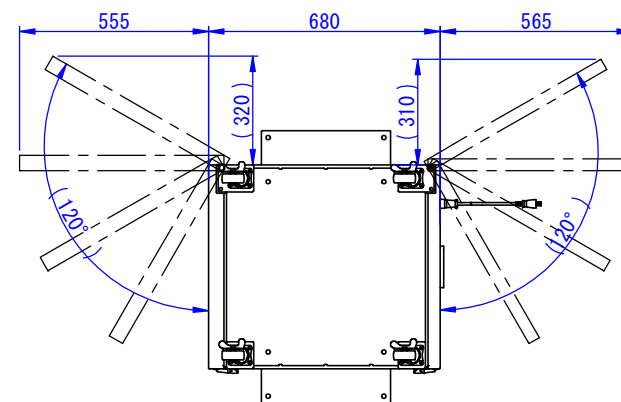
底面
