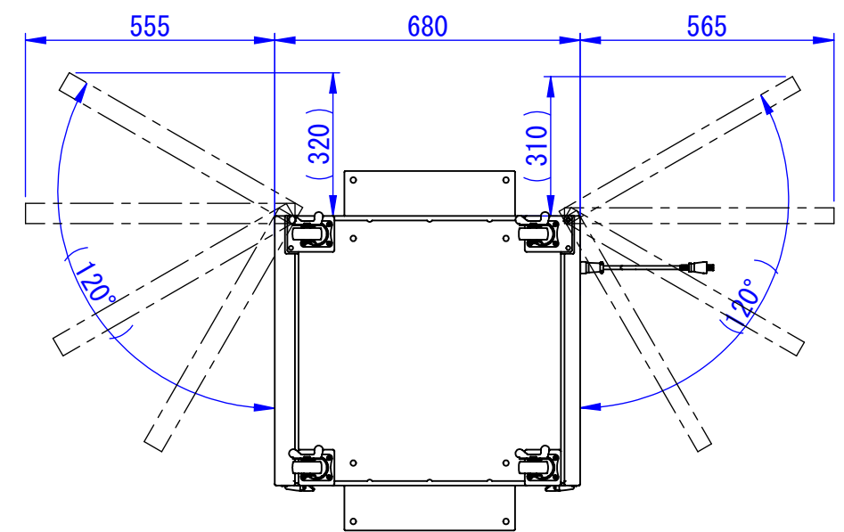
底面
