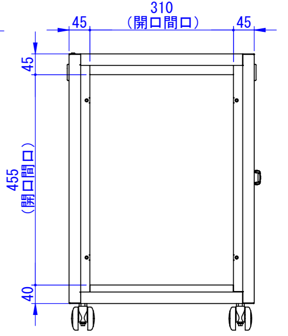
背面 (背面パネルを外した状態)
