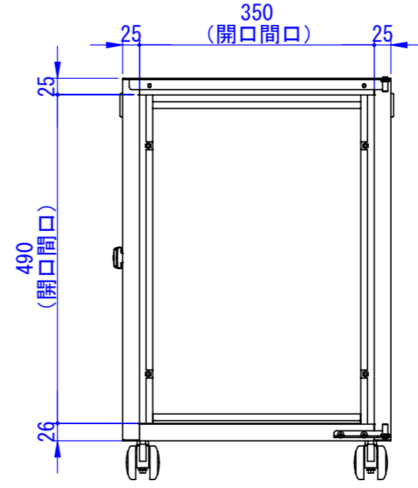
正面 (扉を外した状態)
