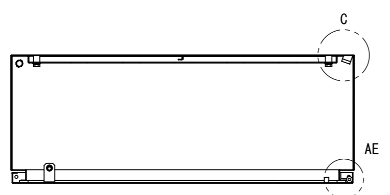
断面図 B-B
