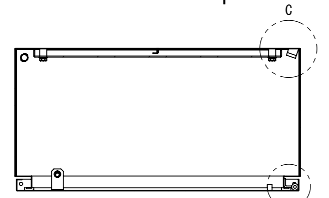
断面図 B-B
