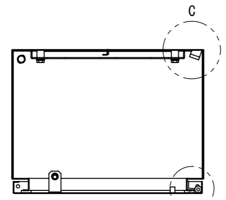
断面図 B-B
