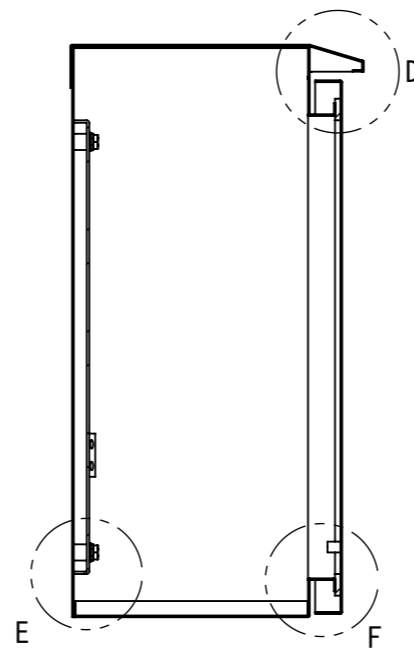
断面図 B-B
