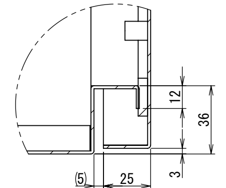
DETAIL AF SCALE 1 : 2
