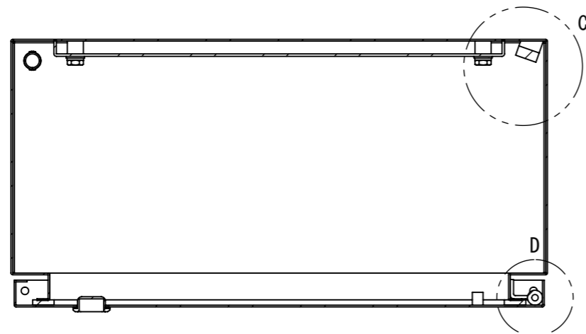
断面図 B-B
