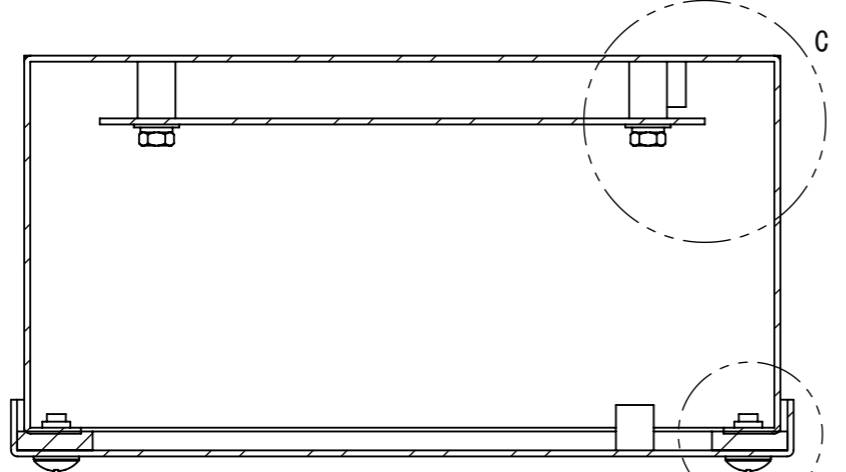
断面図 B-B
