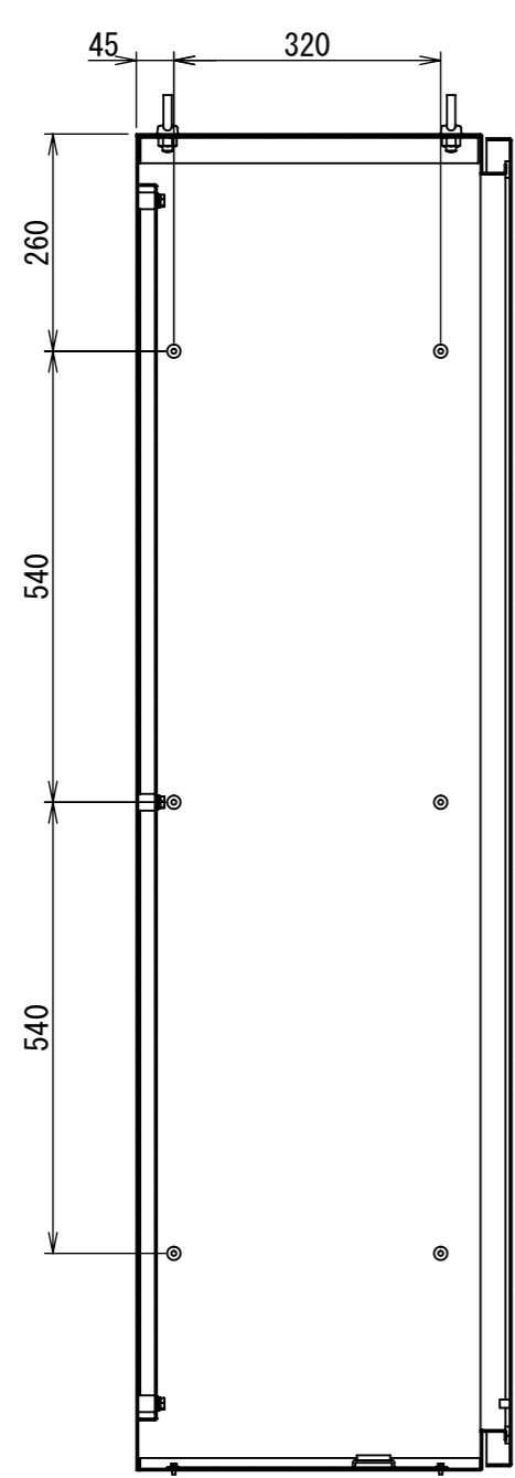
断面図 A-A
