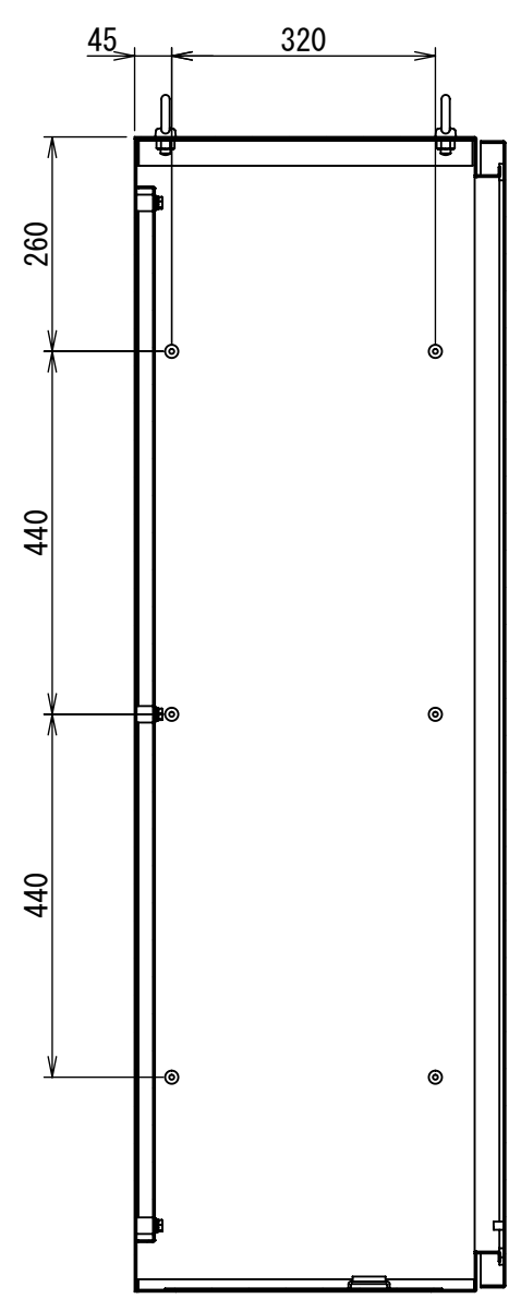
断面図 A-A
