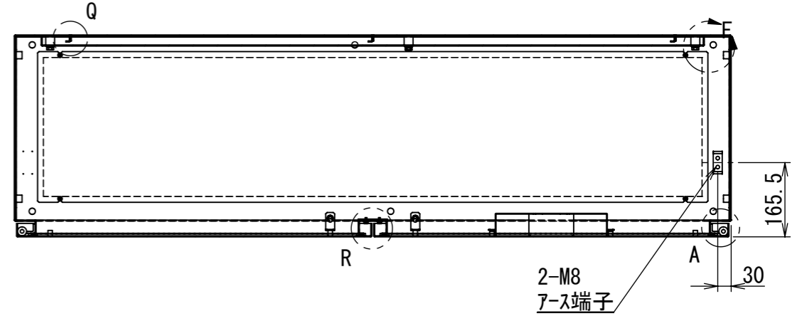
断面図 E-E
