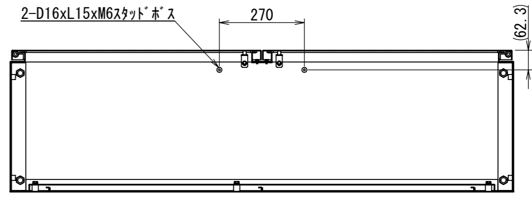
断面図 P-P
