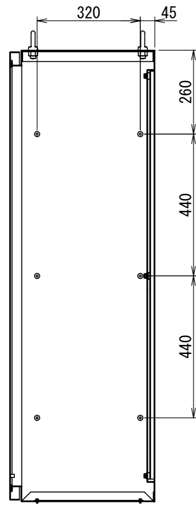
断面図 B-B
