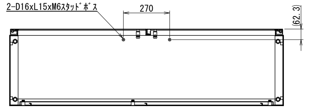
断面図 P-P
