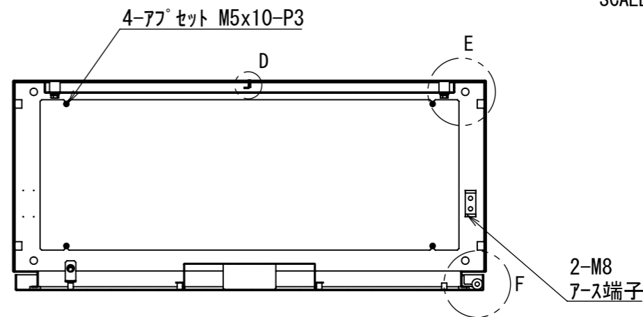
断面図 C-C
