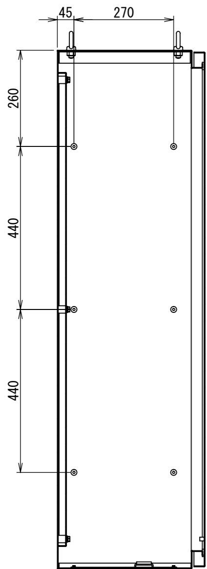
断面図 A-A
