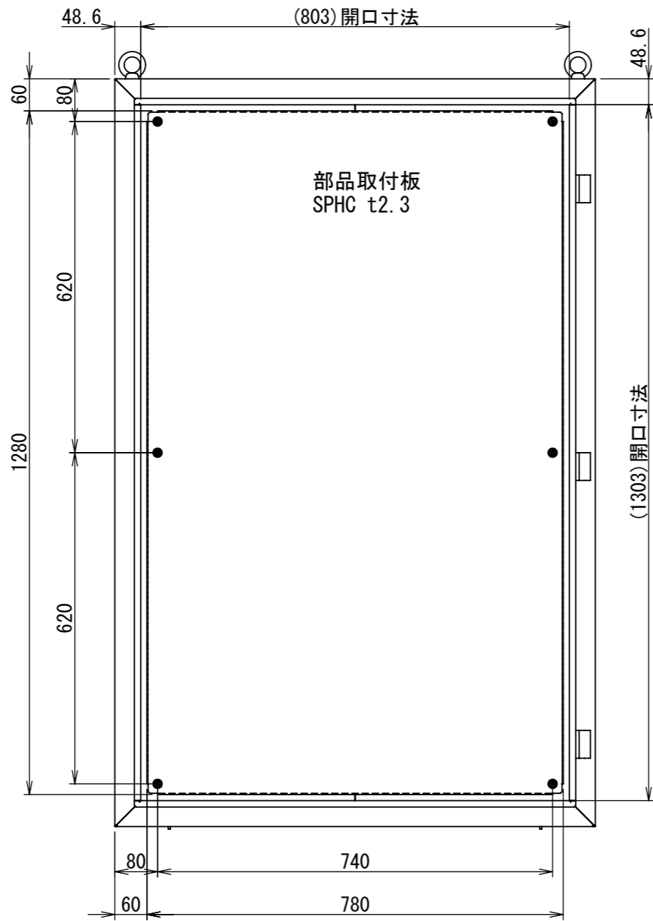
扉開放時
