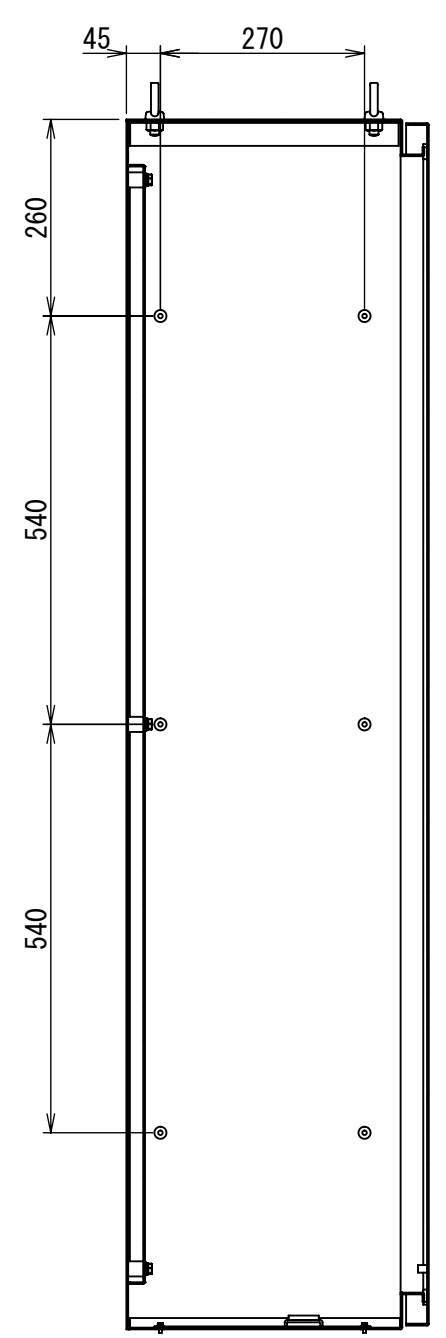
断面図 A-A
