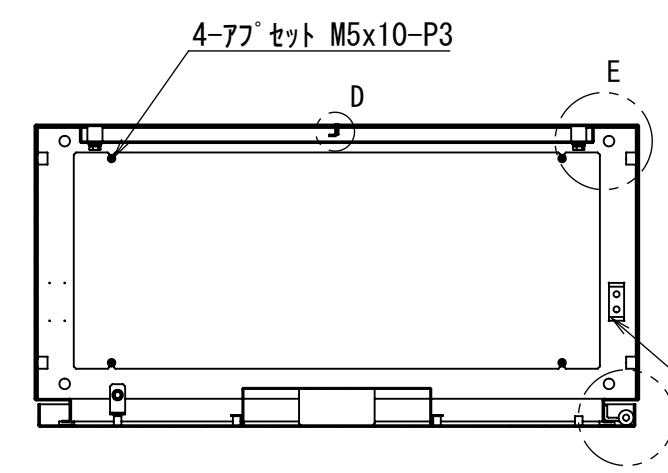
断面図 C-C
