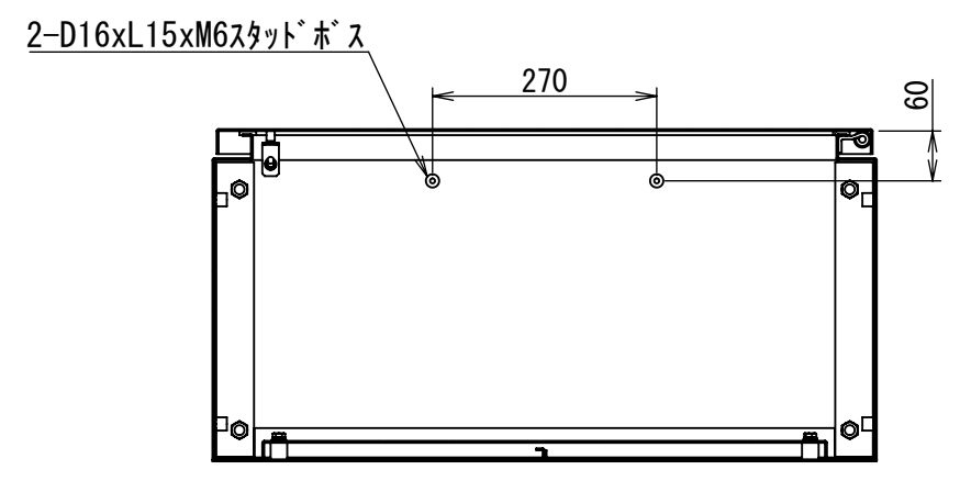
断面図 B-B
