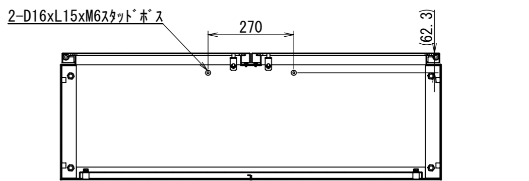
断面図 P-P
