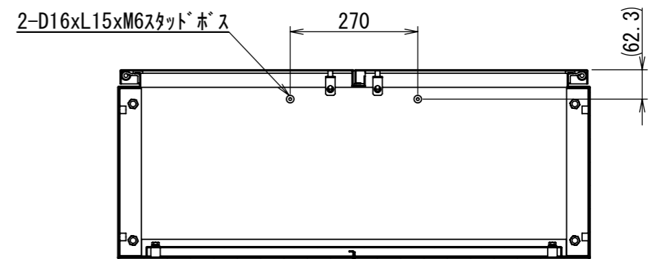
断面図 P-P
