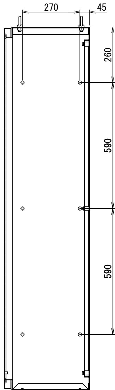
断面図 B-B
