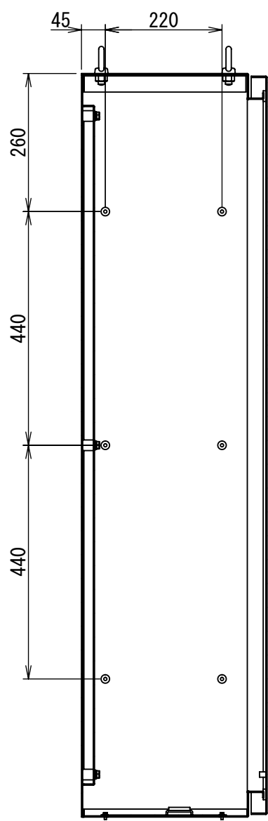
断面図 A-A
