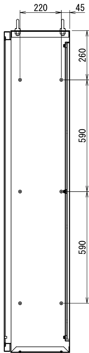
断面図 B-B
