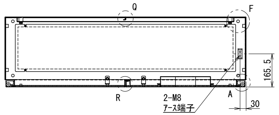
断面図 P-P
