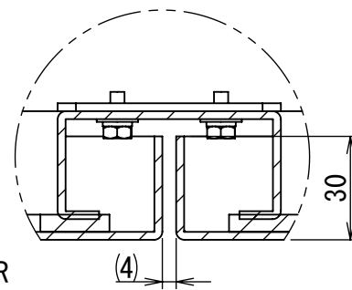
扉開放時
