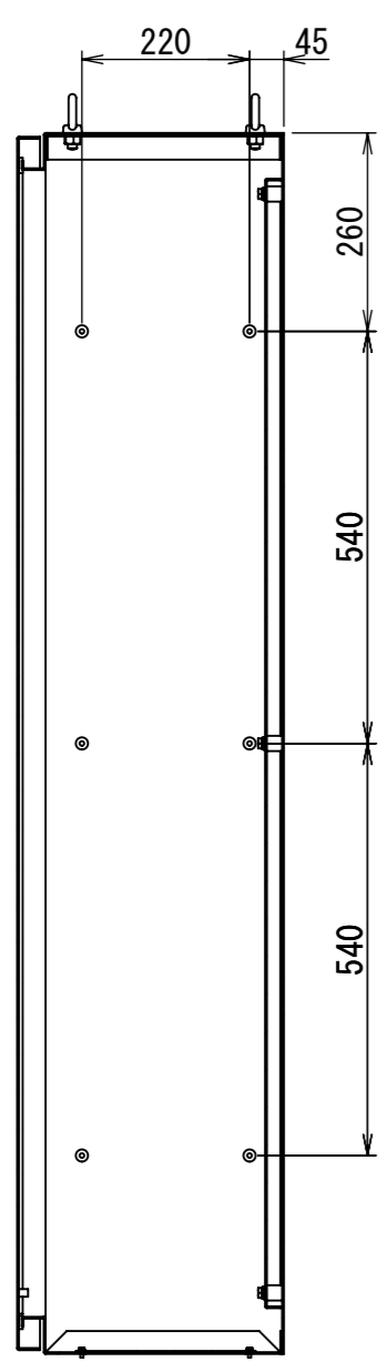
断面図 B-B
