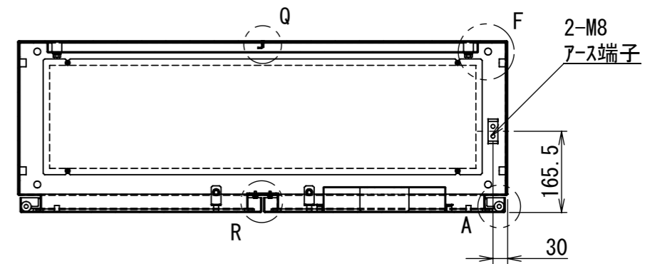
断面図 E-E
