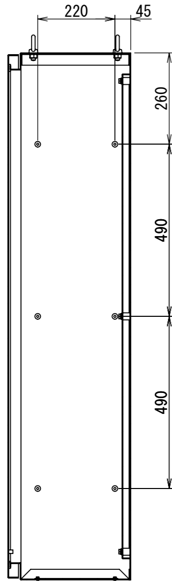
断面図 B-B
